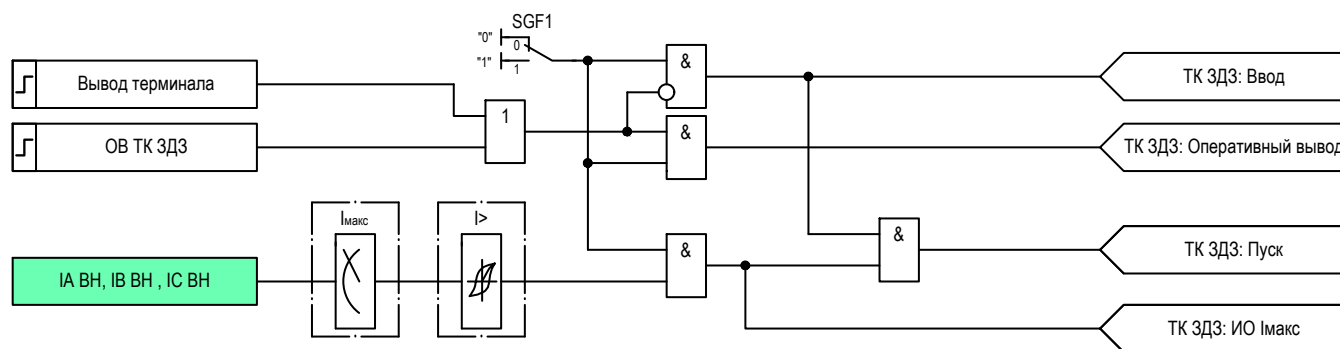
Рисунок 2.16 – Функциональная схема логики ТК 3Д3
