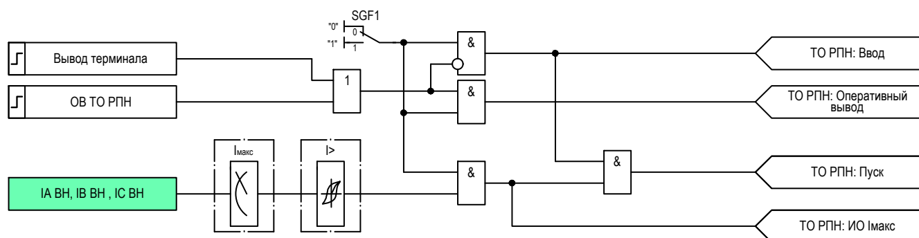
Рисунок 2.17 – Функциональная схема логики ТО РПН
