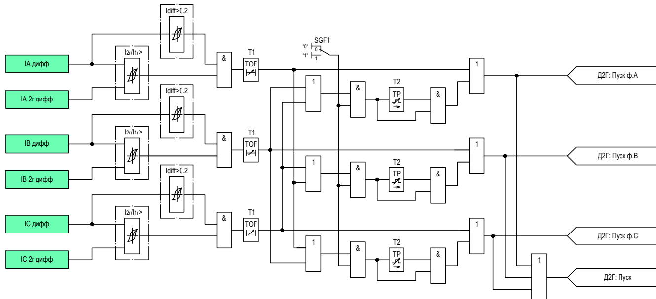
Рисунок 2.5 – Функциональная схема логики Д2Г
