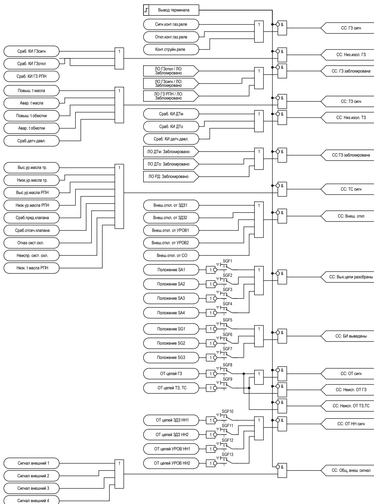
Рисунок 2.32 – Функциональная схема логики сборки сигналов
