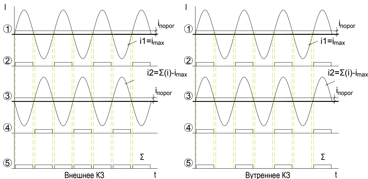
Рисунок 2.7 – Временные диаграммы работы БВКЗ
