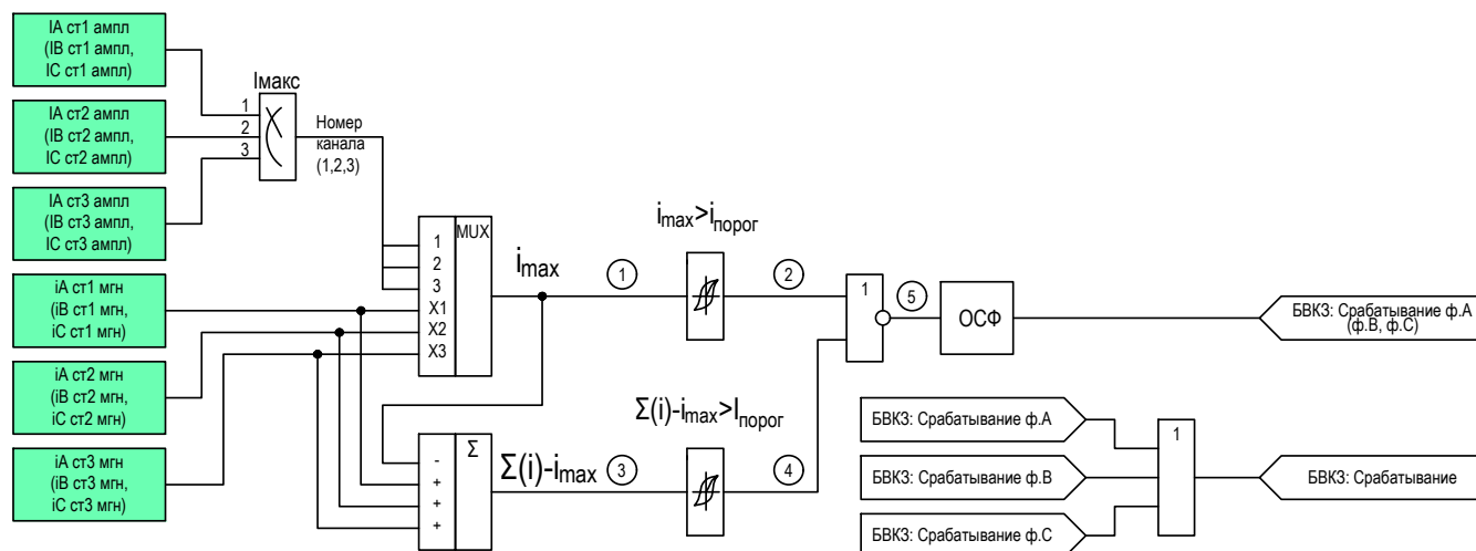
Рисунок 2.8 – Функциональная схема логики БВКЗ
